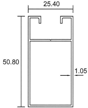
9055B 0.478 Kg/m
