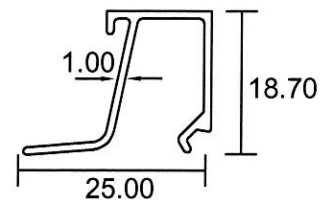
0444N 0.176 Kg/m
