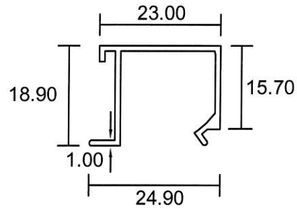
1038 0.190 Kg/m
