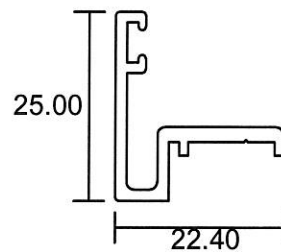
SLF-3508 0.276 Kg/m
