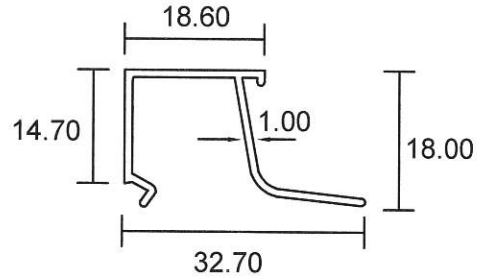
3721 Casement Beading 0.184 Kg/m
