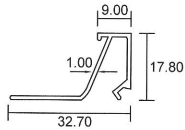
3721L Casement Beading 0.198 Kg/m
