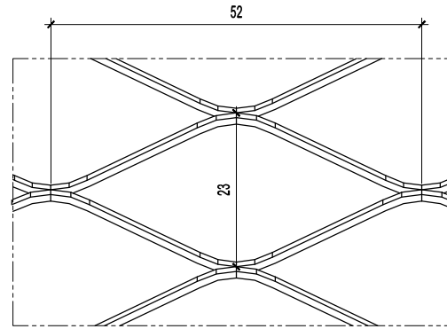
05 DETAIL A SCALE - N.T.S
